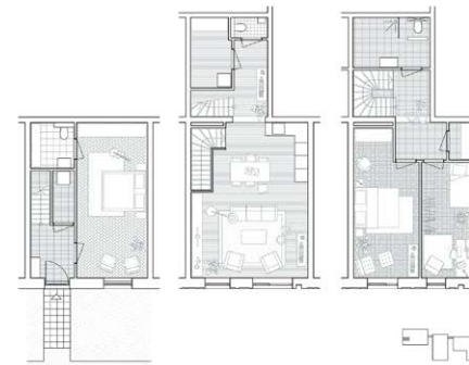
Grondgebonden woning (140m 2 )
