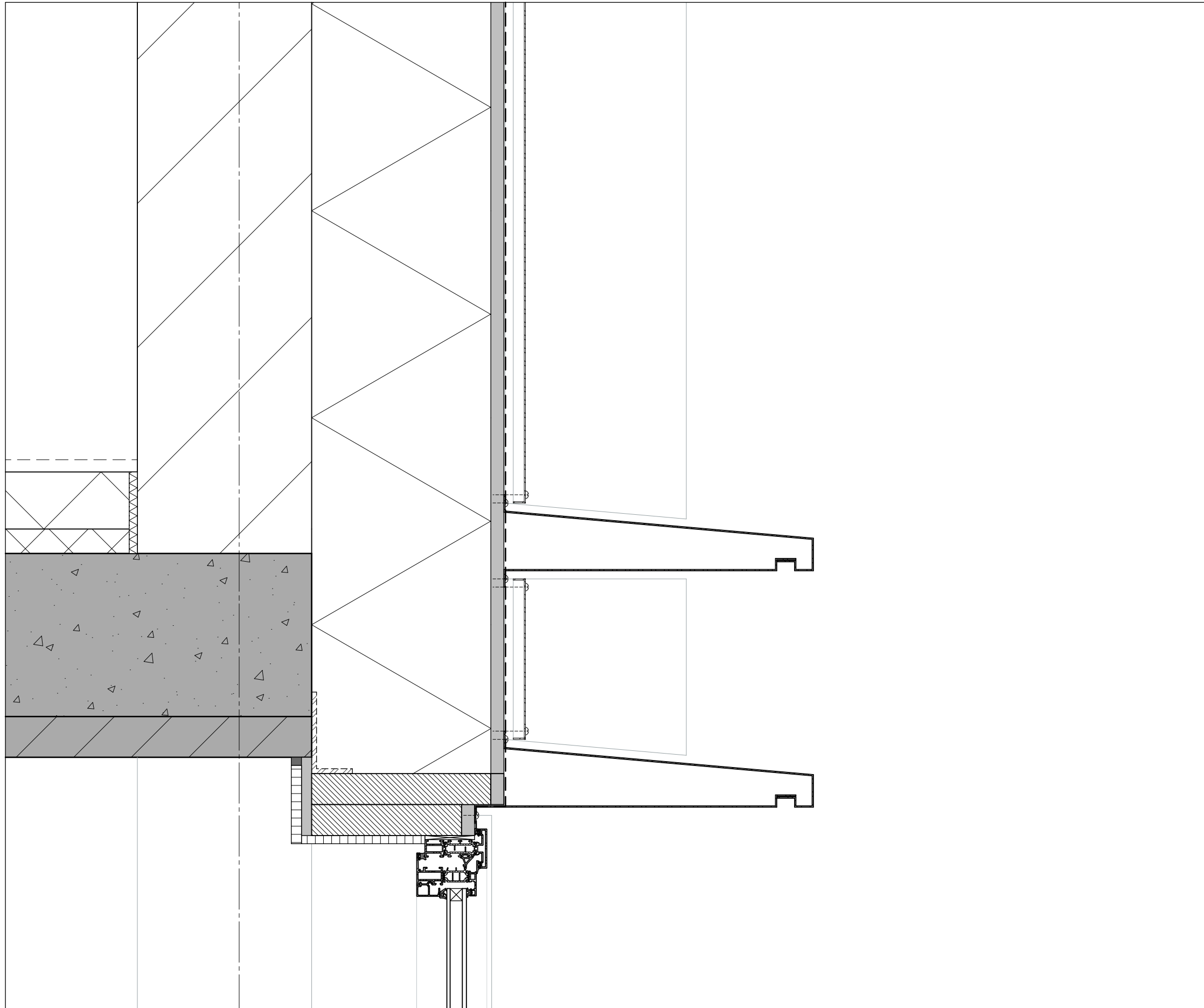
VERTICAAL DETAIL DERDE VERDIEPING - GEVEL SYSTEEM
