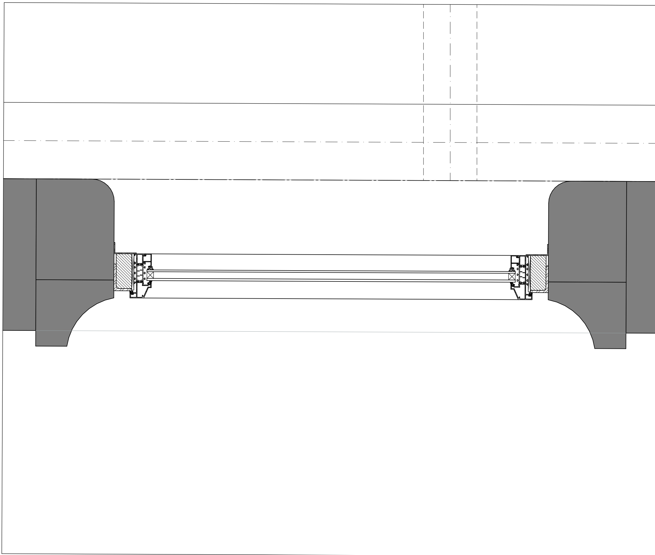
HORIZONTAAL DETAIL EERSTE VERDIEPING - VERDIEPT KOZIJN
