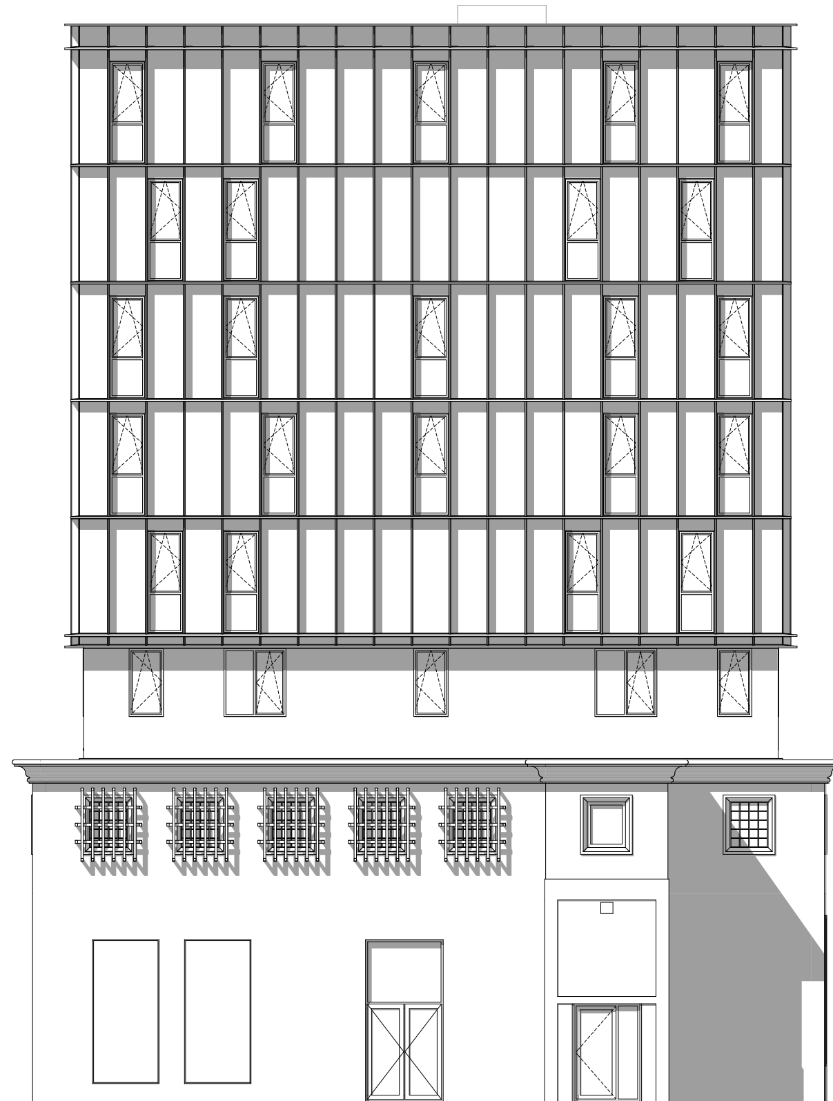
OOSTGEVEL
