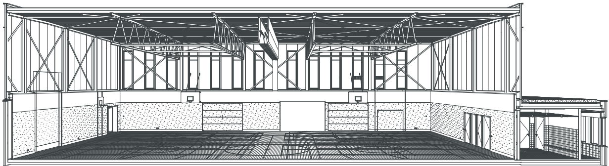
3D doorsnede letterassen
