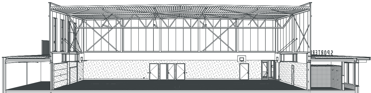
3D doorsnede cijferassen
