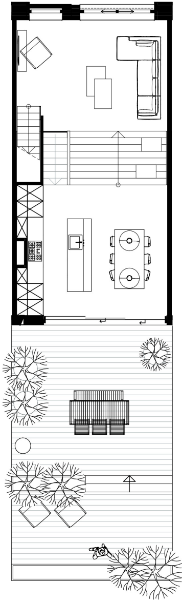
woondek met keuken en woonverdieping
