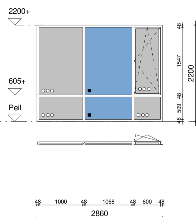
merk A0.08 - aluminium, Reynaers type SL 38 Cubic
