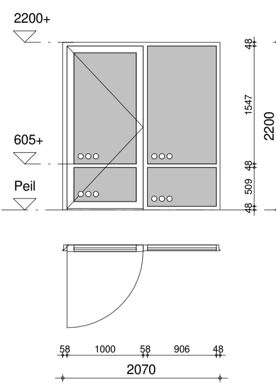
merk A0.03 - aluminium, Reynaers type SL 38 Cubic
