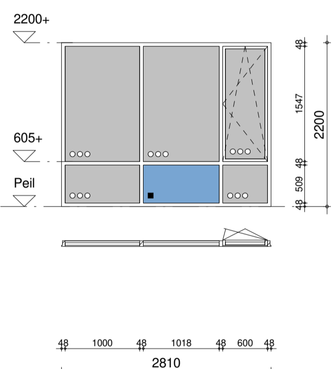
merk A0.09 - aluminium, Reynaers type SL 38 Cubic
