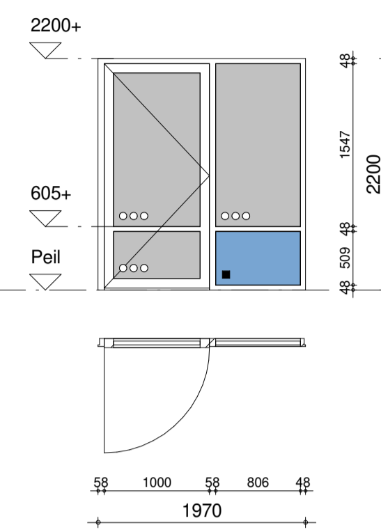
merk A0.04 - aluminium, Reynaers type SL 38 Cubic
