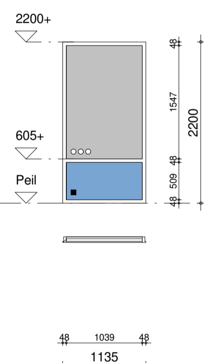
merk A0.07 - aluminium, Reynaers type SL 38 Cubic
