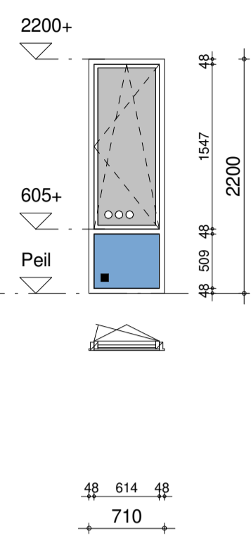
merk A0.02 - aluminium, Reynaers type SL 38 Cubic
