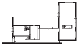
woning type 3 begane grond
